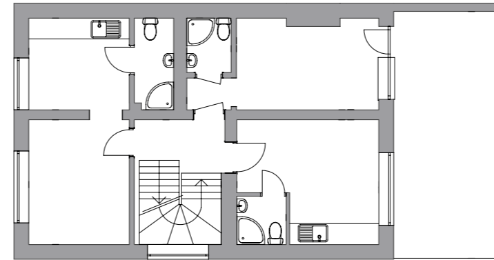
rzut 1. piętra
