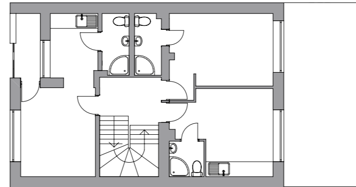
rzut 2. piętra
