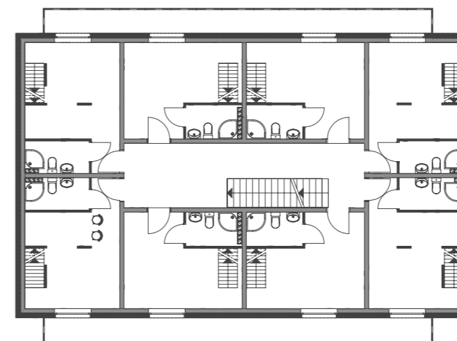
rzut piętra
