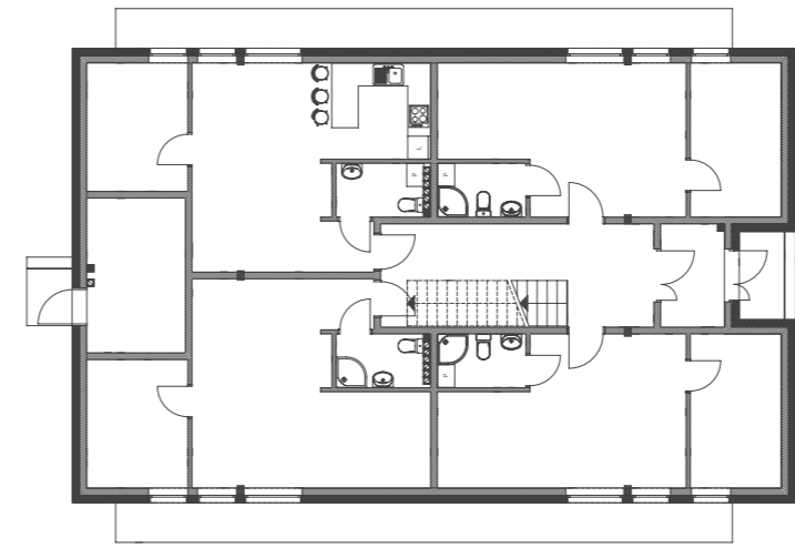
rzut parteru
